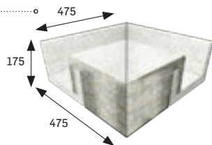
PIEZA ESQUINA EXTERIOR ..... EXTERNAL CORNER PIECE Cod. 901749 [JG745]
